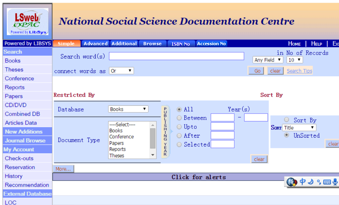
图 2-4 NASSDOC 主页
